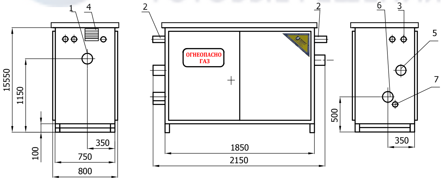
Габаритный чертеж
